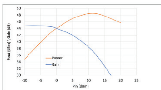
شکل ۶. بهره DCW با TWT دو بخشی [۲۰]
