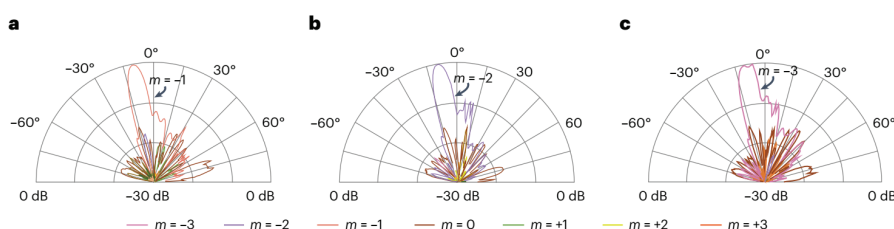
شکل ۱۰: الگوهای تشعشعی اندازه گیری شده در فرکانس‌های هارمونیک مختلف با شکل‌های ۸ و ۹ (به ترتیب از a تا c) [۱]
