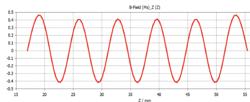
شکل ۱۱. میدان مغناطیسی (۴، T) تولید شده توسط سیستم PPM.
