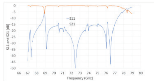
شکل ۱۲. پارامتر S شبیه‌سازی شده از درجه RF [۲۰]
