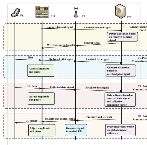
شکل ۲۰- مراحل ارسال و دریافت داده و انرژی در سیستم RIS
