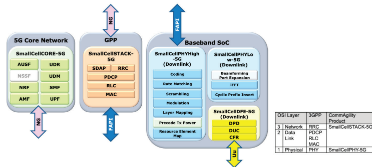
شکل ۲: اجزای نرم افزاری ایستگاه پایه نسل پنجم [۱]
