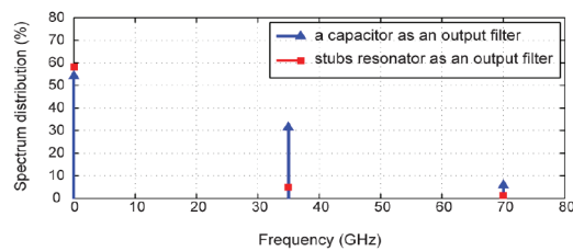
شکل ۵. طیف فرکانسی خروجی یک یکسو کننده از نوع دو برابر کننده
