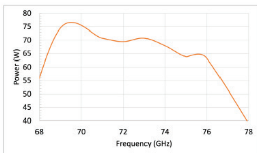
شکل ۵. توان خروجی DCW با TWT دو بخشی [۲۰]
