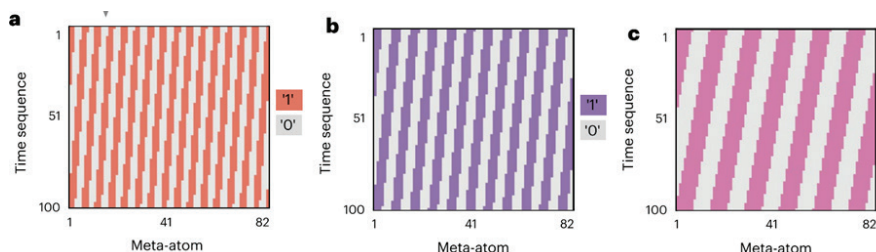
شکل ۵: ماتریس‌های دیجیتال «۰» و «۱» برای تبدیل‌های فرکانس هارمونیک ۱+ با زوایای خروجی (a) 30^\circ ، (b) 10^\circ و (c) 0^\circ درجه [۱]
