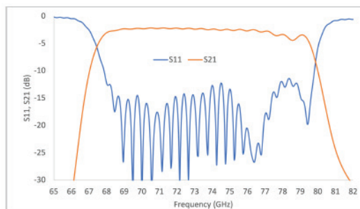
شکل ۹. پارامترهای S برای مدار DCW شکل ۴ [۲۰]
