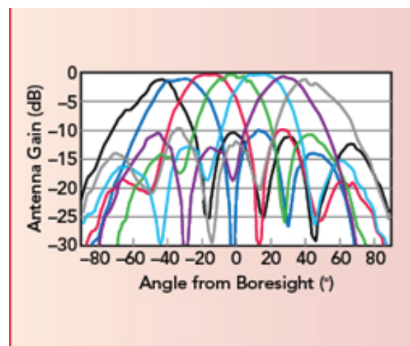
شکل ۲: الگوهای آنتن آرایه‌ای پچ با قطبش عمودی که هدایت پرتو را بین زوایای +۴۵ و -۴۵ درجه نشان می‌دهد [۱]
