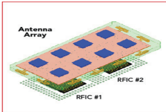
شکل ۴: تراز گرهای RFIC به سمت پشت بردی که شامل آرایه های آنتن است، نصب می شوند [۱]
