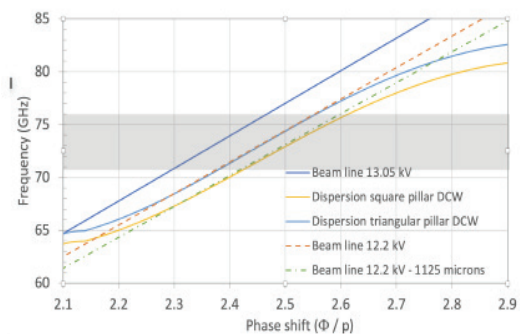
شکل ۲. پراکنده‌گی ۱۸ DCW با ستون مثلثی به عنوان تابعی
