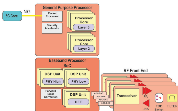
شکل ۲: یک gNodeB یکپارچه شامل یک هسته 5G، PHY، DFE، فرانت اند RF، و پردازش پکت لایه ۲ و لایه ۳ [۱]
