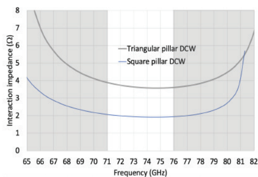
شکل ۳. امیدانس اثر متقابل DCW با ستون مثلثی و DCW با ستون
