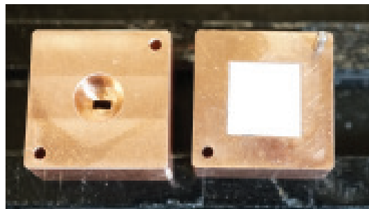
شکل ۲۶. بلوک‌های دریچه RF، حفره (چپ)، صفحه آلومینیومی (سمت راست) [۲۰]
