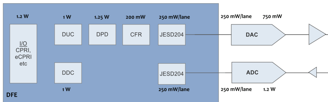
شکل ۴: مصرف توان بر حسب کارکرد در یک ترنسپور گسیسته 5G [۲]
