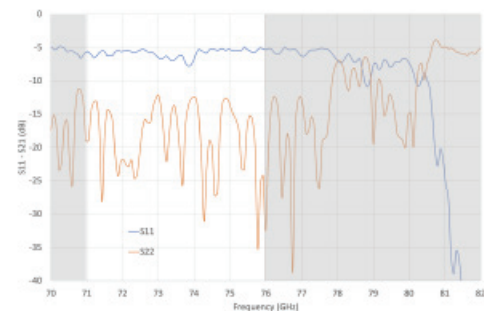
شکل ۲۵. پارامترهای S اندازه‌گیری شده مدار DCW پس از پیوند نفوذی [۲۰]
