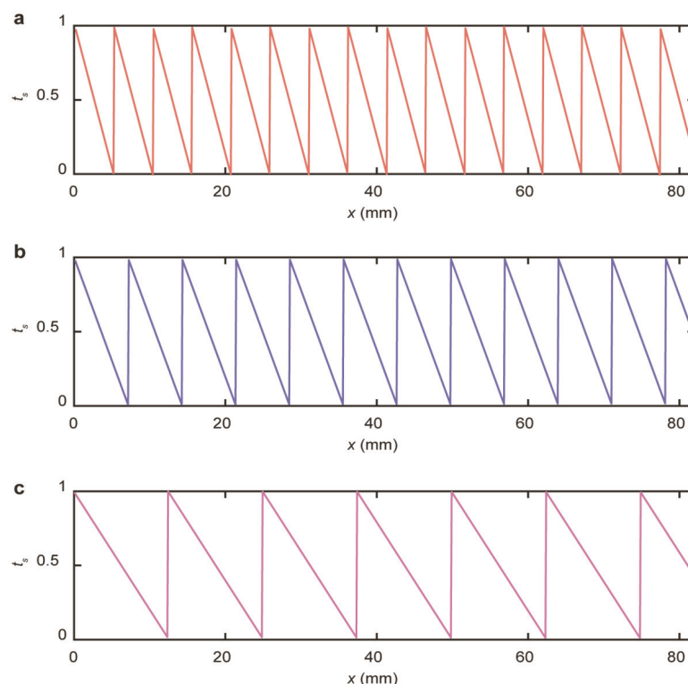
شکل ۴: شیفت های زمانی نرمالیزه مورد نیاز برای تبدیل فرکانسی، (a) معادل با زاویه خروجی ۵۰°، (b) ۱۰° و (c) ۳۰° درجه [۱]
