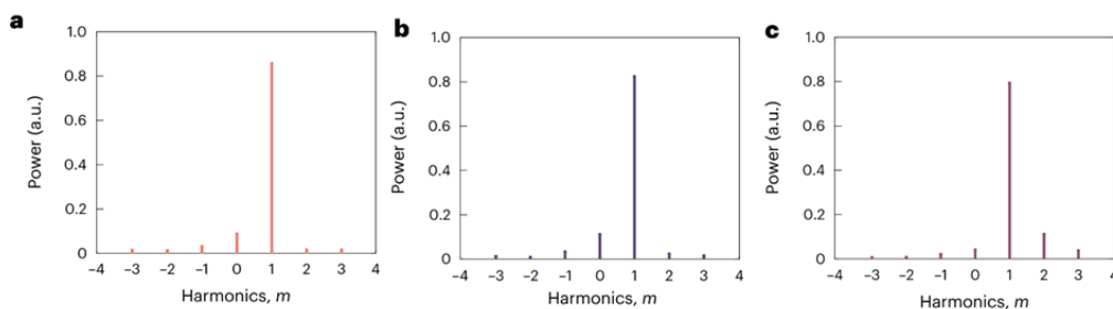
شکل ۶: توزیع‌های توان اندازه‌گیری شده در هارمونیک‌های مختلف معادل با ماتریس‌های شکل ۵ (به ترتیب از a تا c) [۱]
