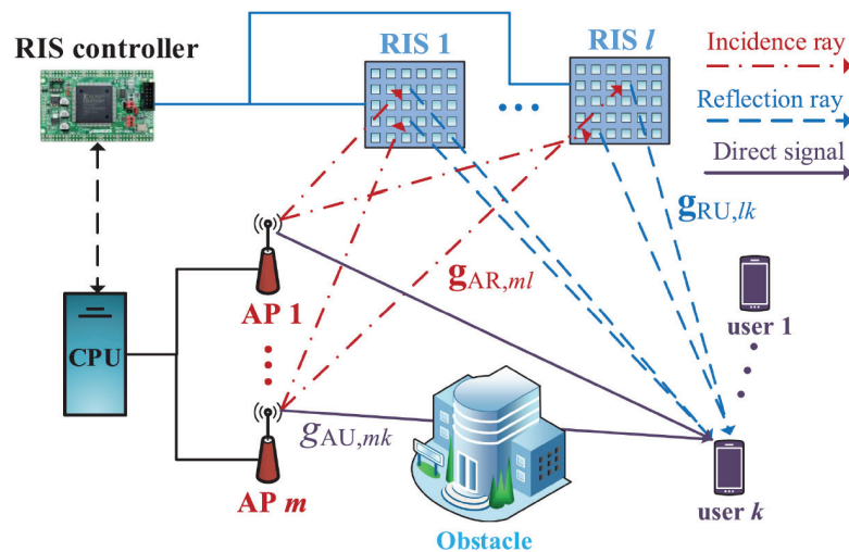
شکل ۱۹- استفاده از فناوری RIS در یک شبکه CFmMM [۹]
