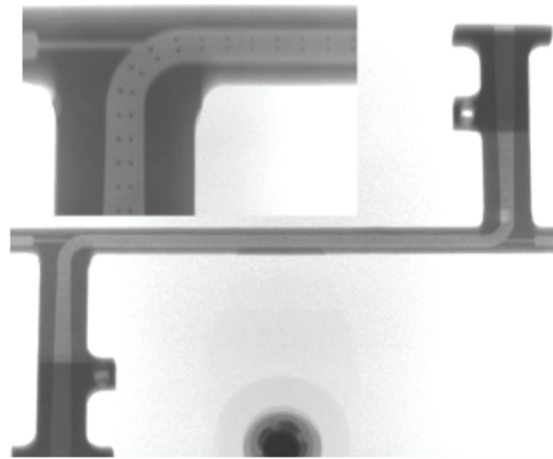
شکل ۲۴. تصاویر سی‌تی اسکن اشعه ایکس از مدار DCW متصل شده. (بالا) جزئیات خم، (پایین) مدار DCW کامل [۲۰]
