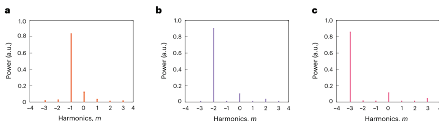
شکل ۹: توزیع‌های توان اندازه‌گیری شده در هارمونیک‌های مختلف برای تبدیل‌های فرکانسی هارمونیک m = -1, -2, -3 معادل شکل ۸
