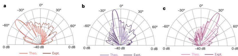
شکل ۷: الگوهای تشعشعی محاسبه شده بر اساس تئوری و اندازه‌گیری شده در فرکانس هارمونیک ۱+ معادل با شکل‌های ۵ و ۶ (به ترتیب از a تا c) [۱]
