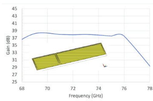
شکل ۱۰. بهره DCW با TWT دو بخشی [۲۰]
