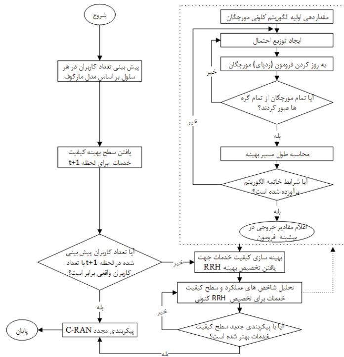
شکل ۳- الگوریتم پیکربندی C-RAN بر اساس مدل مارکوف و کلونی مورچگان [۱]
