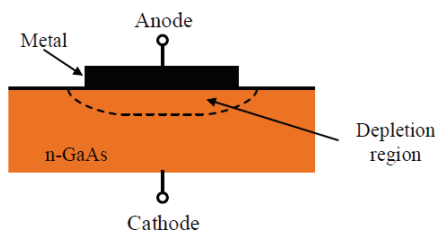
شکل ۲. یک اتصال شاتکی [۷]
