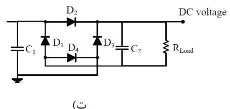
شکل ۴. چند طراحی معروف یکسو کننده بر پایه دیود شاتکی.
