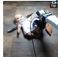
MolmoAct2 (VLA)
