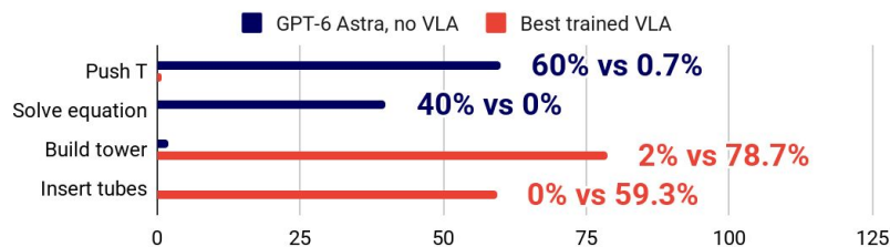
GPT-6 Astra
