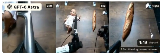
GPT-6 Astra
